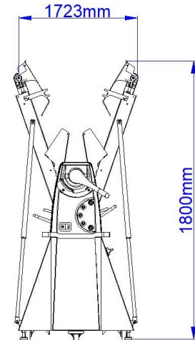
VISTA FRONTAL 2
