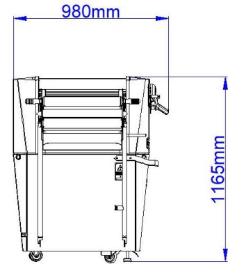
VISTA LATERAL
